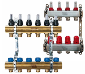
Коллекторные узлы
